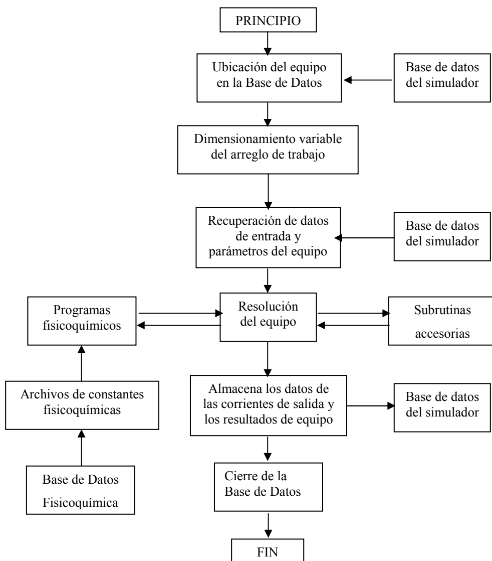
Figura 7: Esquema de cálculo de cada módulo o equipo del simulador
