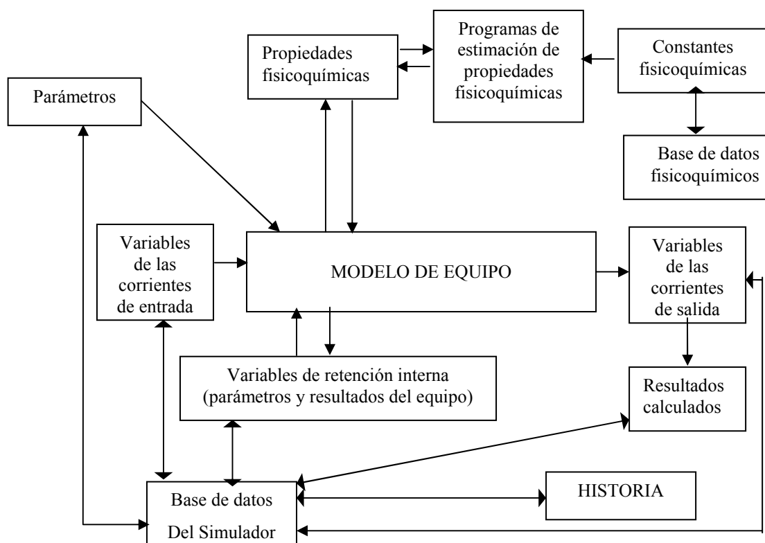
Figura 6: Arquitectura típica de un simulador modular secuencial
